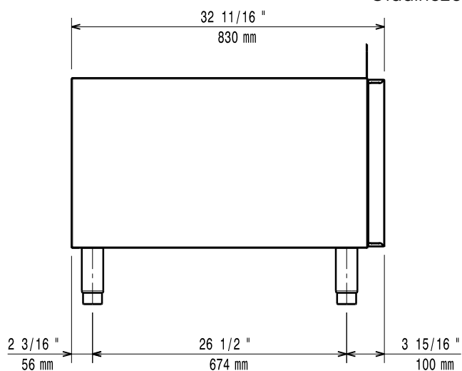
Oldalnézet
